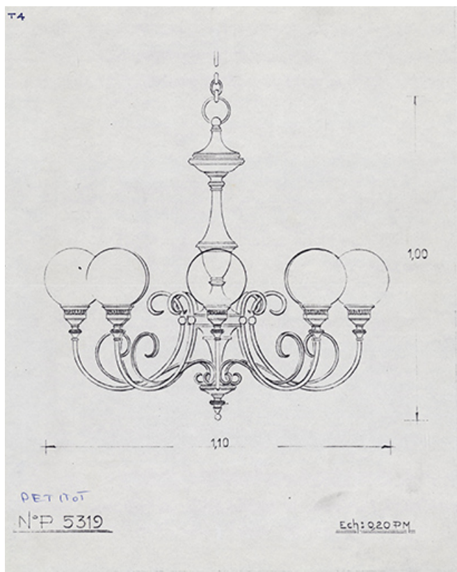
[Lustrerie spéciale]. N° P. 5319. S.d. [1980].
