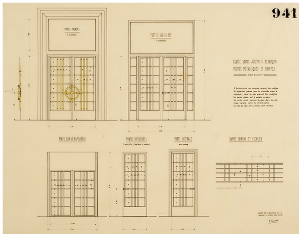
Dessin des portes de l'église Saint-Joseph à Besançon. Juillet 1954. 25, Besançon, 18 avenue Villarceau
