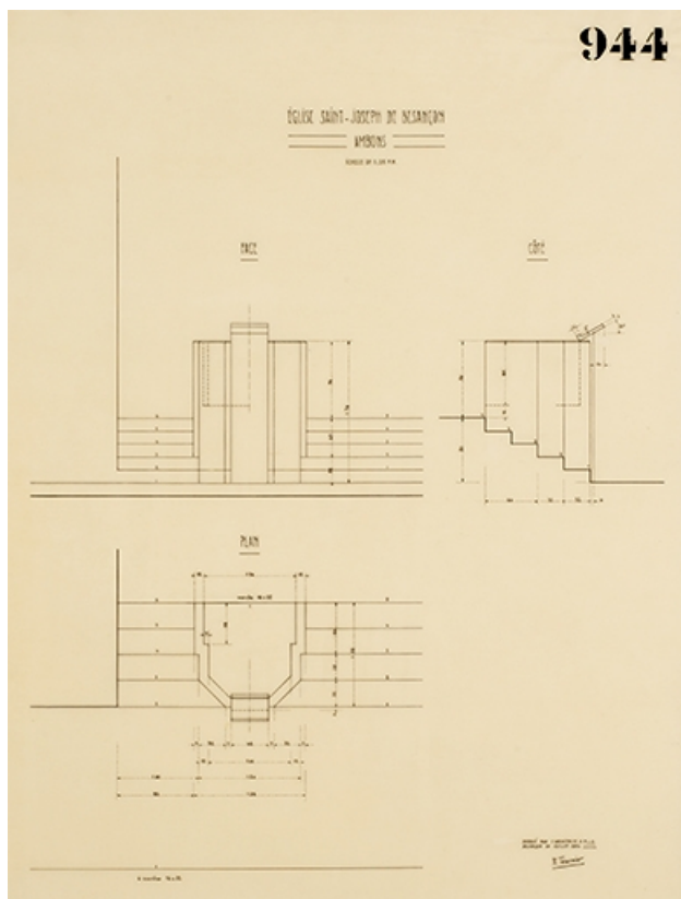
Plan et élévations des ambons de l'église Saint-Joseph. Juillet 1954. 25, Besançon, 18 avenue Villarceau
