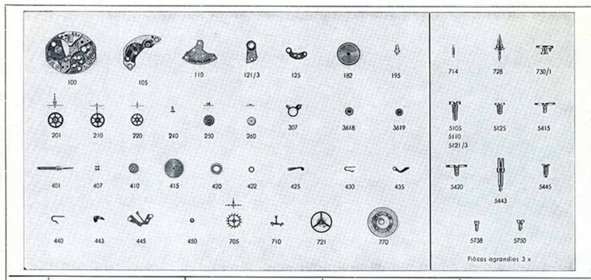
Calibre 5 1/2''' 68 - 17 rubis [éclaté des fournitures], 1973. 25, Maîche
