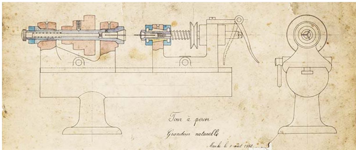
Tour à percer. Grandeur naturelle, 5 août 1912.
