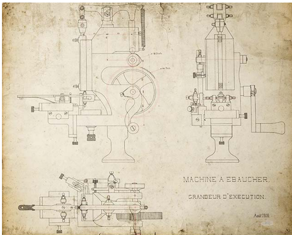
Machine à ébaucher. Grandeur d'exécution, août 1916.
