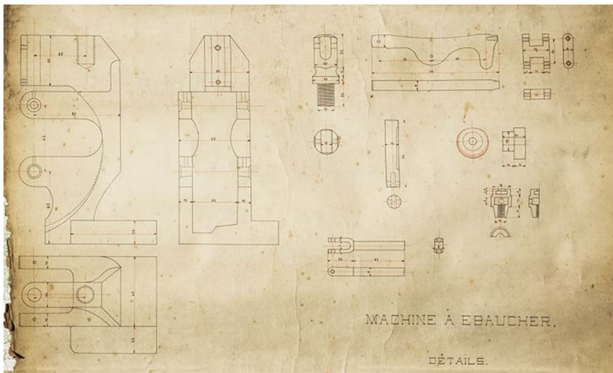
Machine à ébaucher. Détails, 1916.
