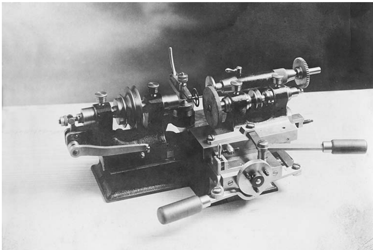
[Machine à rectifier les siettes ?], 2e quart 20e siècle ? (après 1936). 25, Maîche, 13 rue Sous Montjoie
