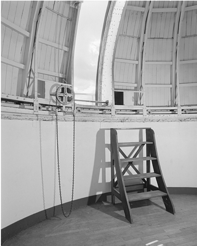
Vue d'ensemble du système d'ouverture du dôme.
