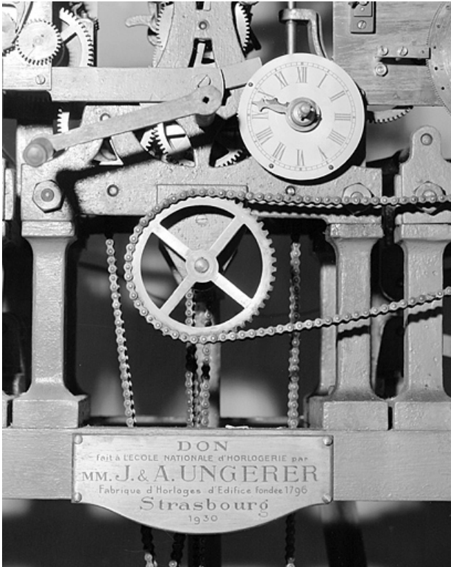
Cadran de contrôle et plaque.
