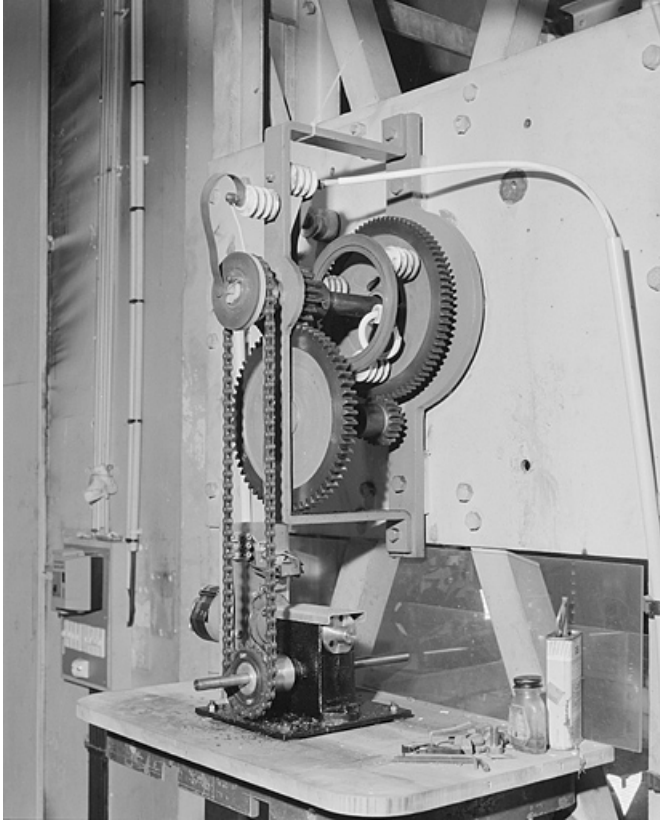
Le système d'entraînement des aiguilles.
