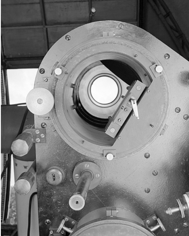
Partie oculaire d'une des deux lunettes photographiques.
