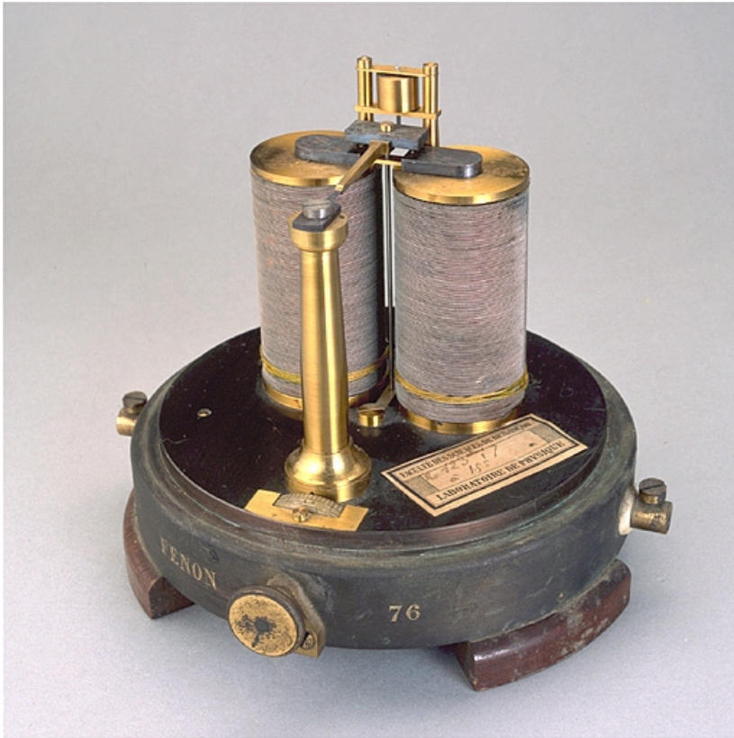
Le relais à deux bobines n° 76.
