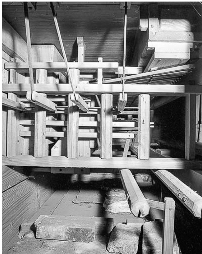
Mécanique des rouleaux de registre vue de face.
