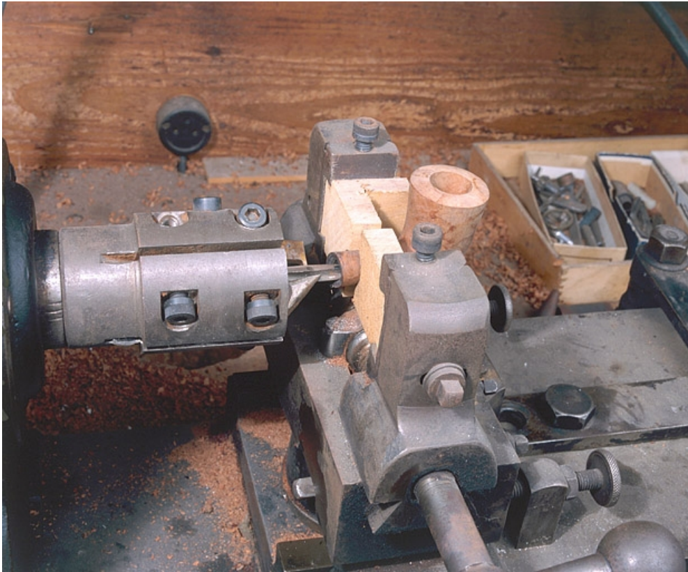
Le mandrin pénètre dans la tige pour la chanfreiner (atelier principal).
