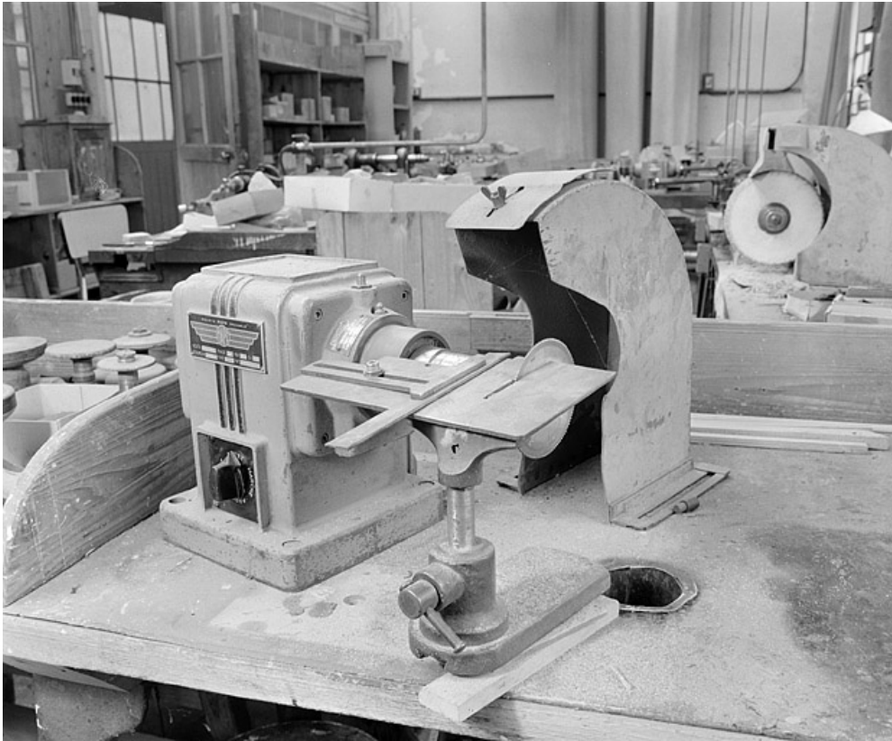
Vue d'ensemble de la scie (atelier de finissage). 25, Baume-les-Dames rue des Pipes, lieudit : Gondé
