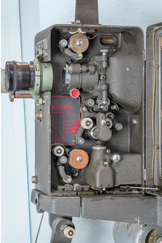
Mécanisme projecteur (système d'entraînement du film et objectif). 21, Lacanhe rue de l' Église
