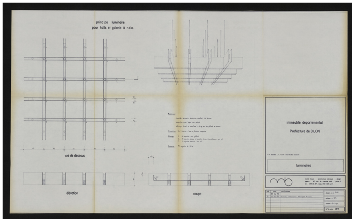
Elévation perspective, plan et coupe des luminaires, 15 février 1979. Boyer, Michel (architecte d'intérieur) (Archives départementales de la Côte-d'Or, Dijon, 32 J 106)
