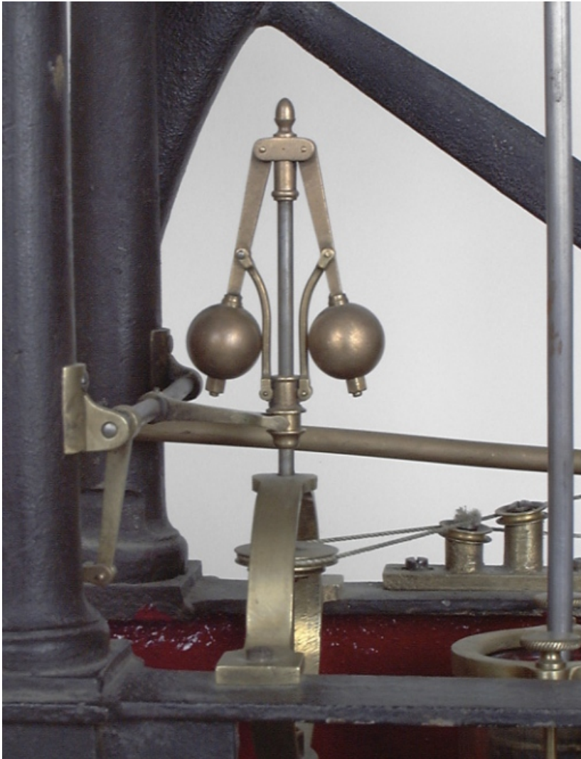
Détail du régulateur à boule.
