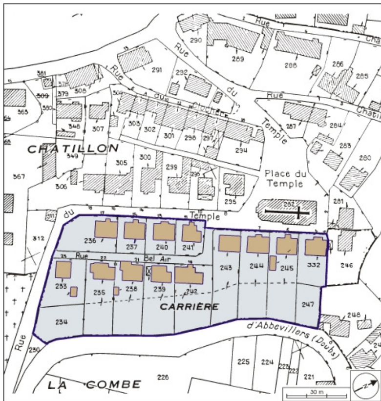
Plan-masse et de situation. Extrait du plan cadastral, 1979, section AH, 1:1000. 90, Beaucourt, lieudit : cité du Temple
