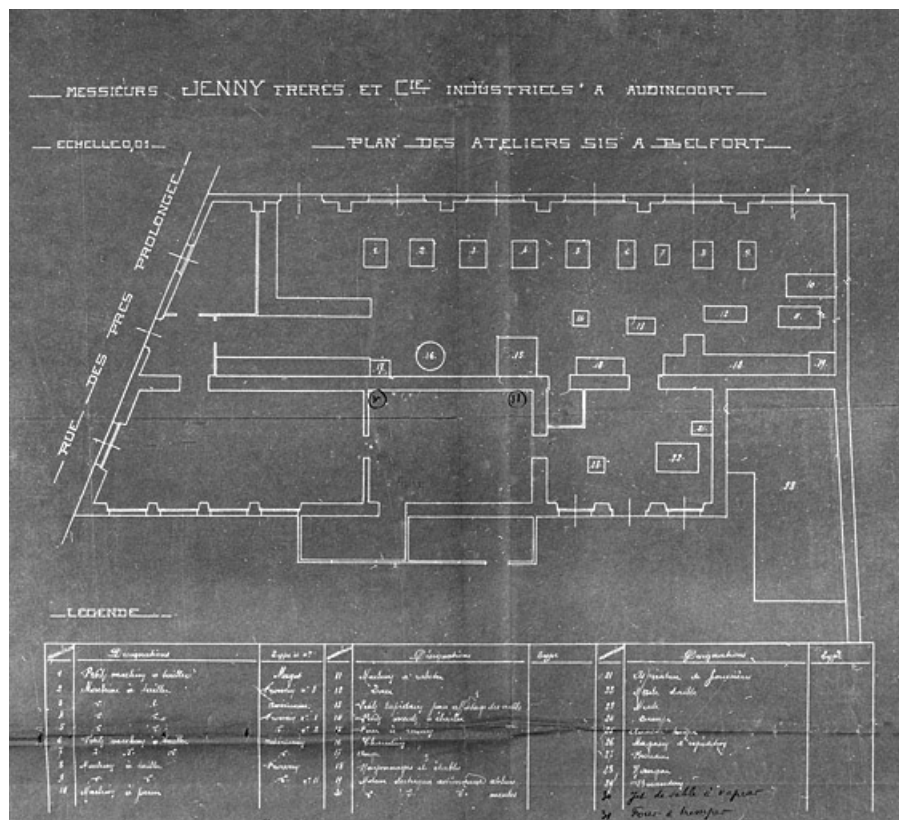
Messieurs Jenny frères et Cie, industriels à Audincourt. Plan des ateliers sis à Belfort. 90, Belfort, 2 rue Jules Ferry
