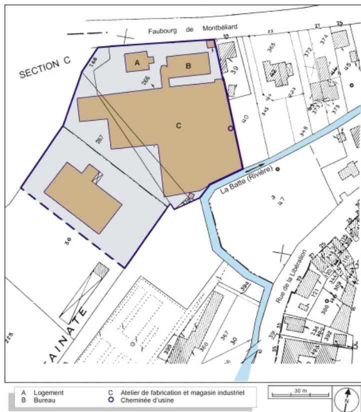
Plan-masse et de situation. Extrait du plan cadastral, 1984, section AI, 1:1000. 90, Delle, 37 faubourg de Montbéliard
