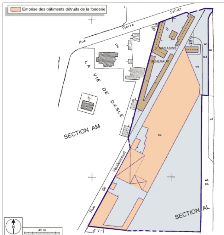
Plan-masse et de situation. Montage d'extraits de plan cadastral, 1979, sections AL et AM, 1:000, le tout réduit à 1:1500. 90, Beaucourt rue de Vaudoncourt
