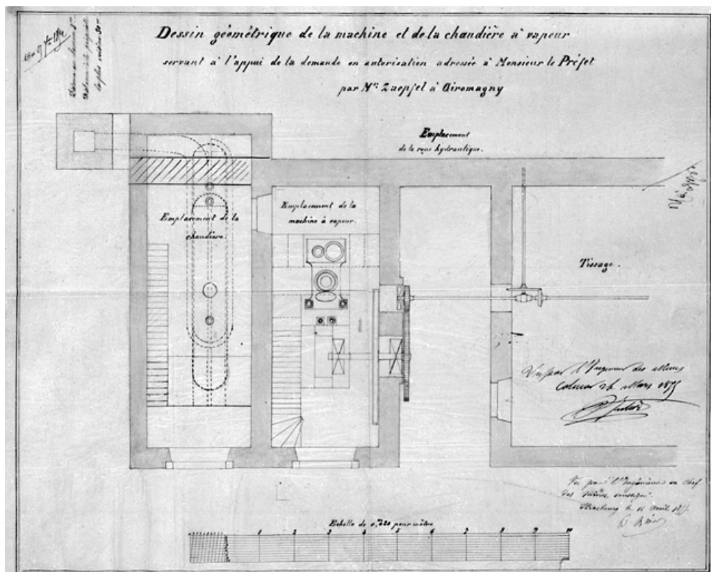
Dessin géométrique de la machine et de la chaudière à vapeur servant à l'appui de la demande en autorisation adressée à Mr le préfet par M. Zoeffel à Giromagny.
