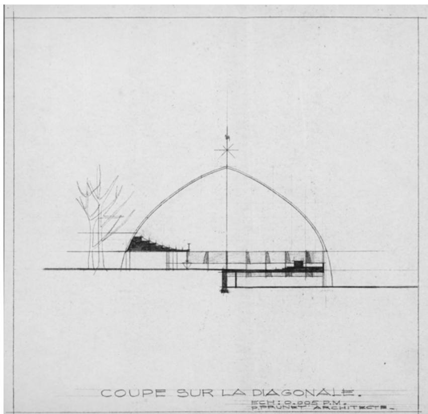
Coupe sur l'axe diagonal de l'église Sainte-Thérèse des Rosoirs.
