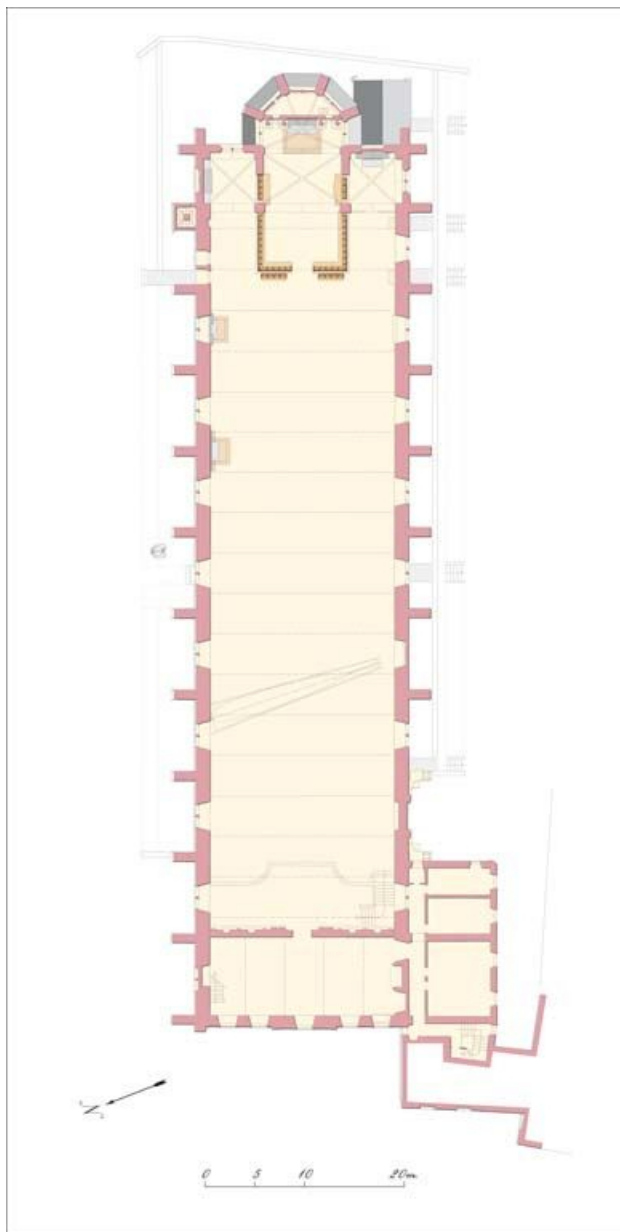
Plan régulier du rez-de-chaussée, niveau supérieur.
