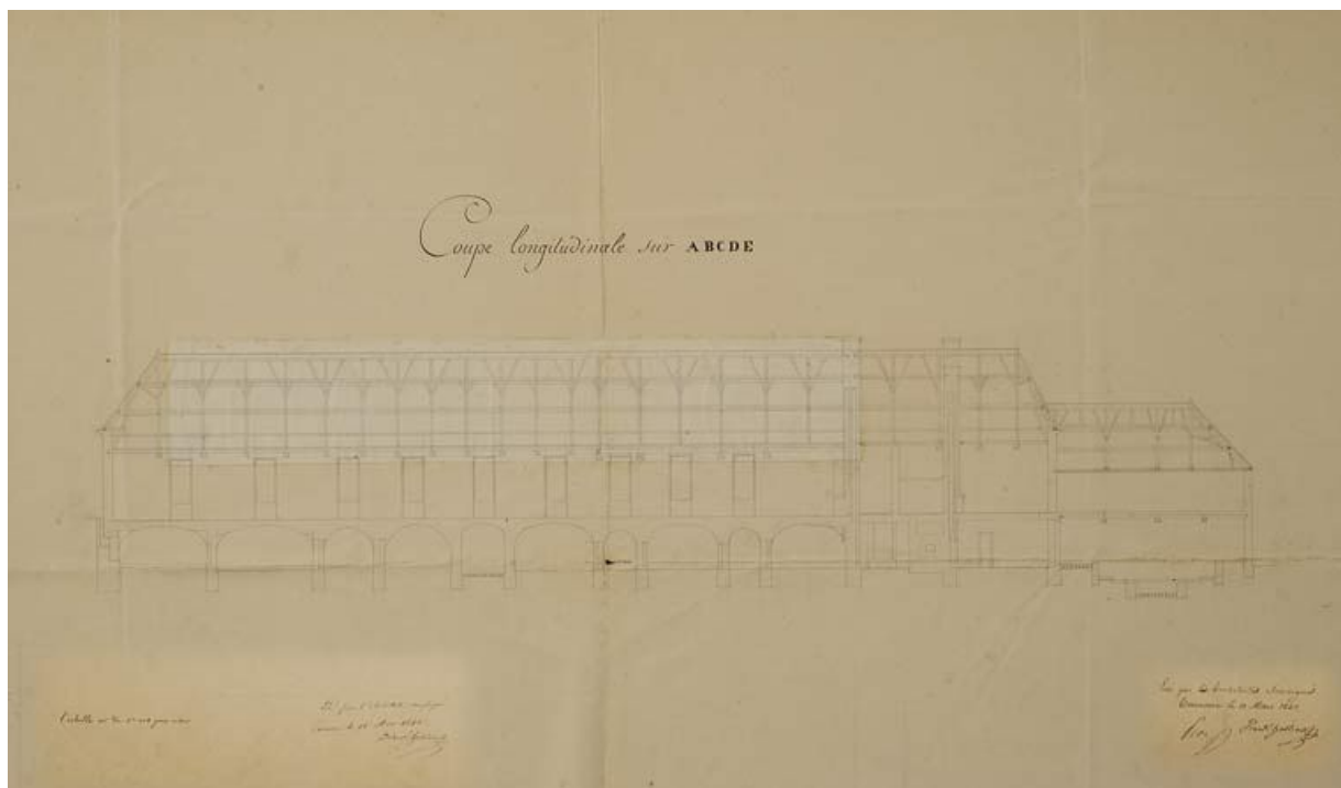
Projet d'un nouvel hôpital par emploi des greniers et salle de la Reine (1840). 89, Tonnerre Hôpital
