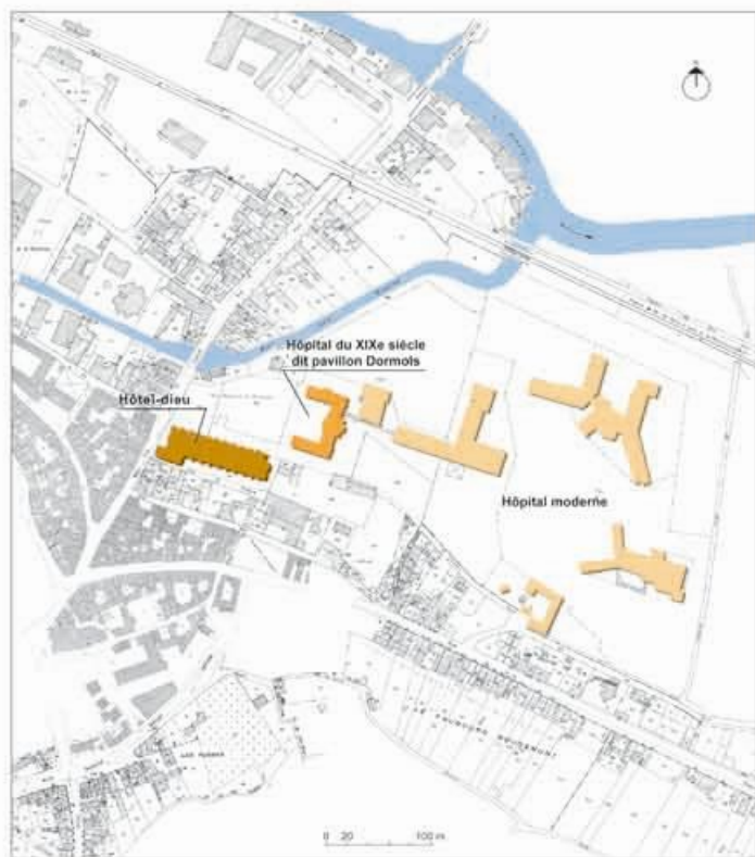
plan masse de l'ensemble hospitalier, extrait du plan cadastral au 1/1000e réduit au 1/4000e 89, Tonnerre Hôpital
