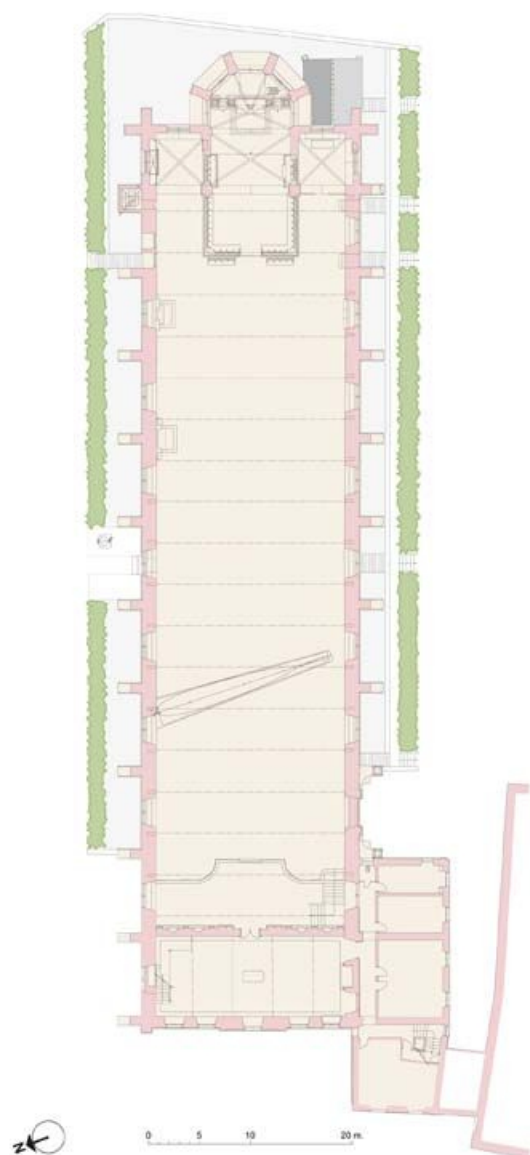
plan au 1/500 du niveau supérieur, dessin sous AutoCad d'après un relevé régulier de 2004 89, Tonnerre Hôpital
