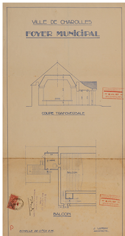
Ville de Charolles. Foyer municipal. Coupe transversale [et] Balcon. S.d. [Visa du 16 avril 1937]. 71, Charolles, 40B rue Baudinot
