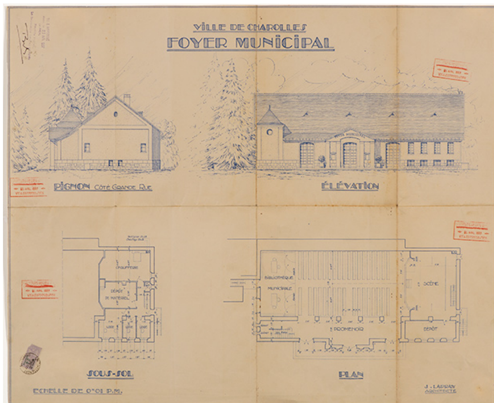
Ville de Charolles. Foyer municipal. Plan d'ensemble [plans et élévations]. S.d. [Visa du 16 avril 1937]. 71, Charolles, 40B rue Baudinot
