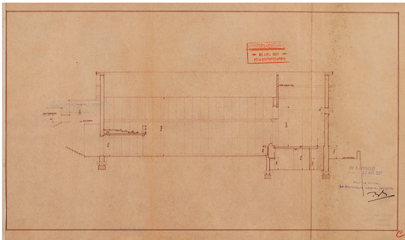
Ville de Charolles. Foyer municipal. Coupe longitudinale. S.d. [Visa du 16 avril 1937].
