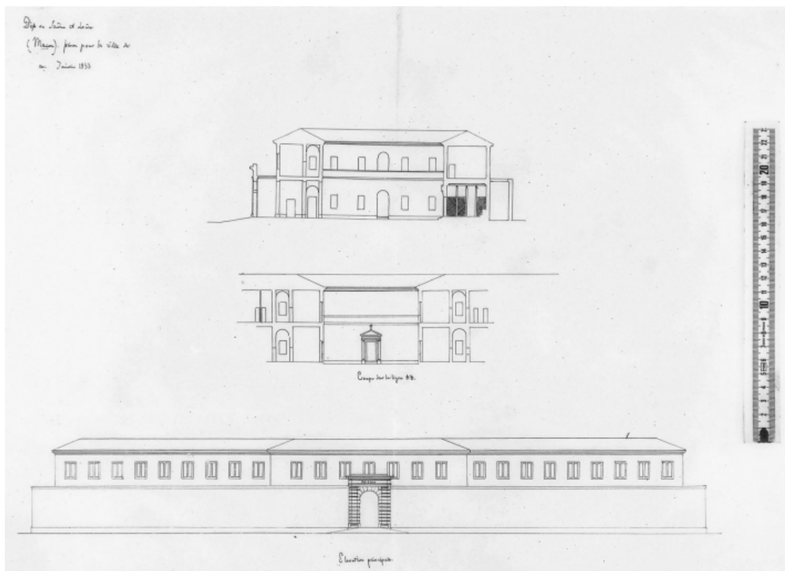
Projet d'extension (élévation et coupes). 1833.
