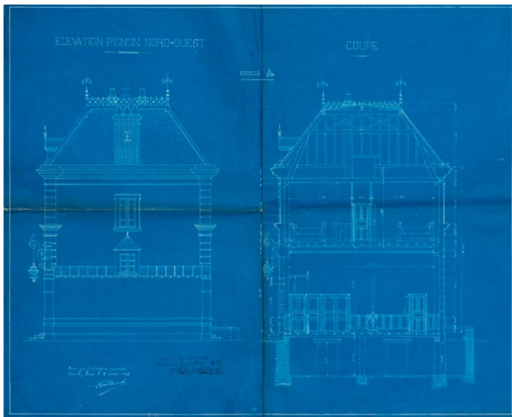
Élévation de la façade latérale et coupe.
