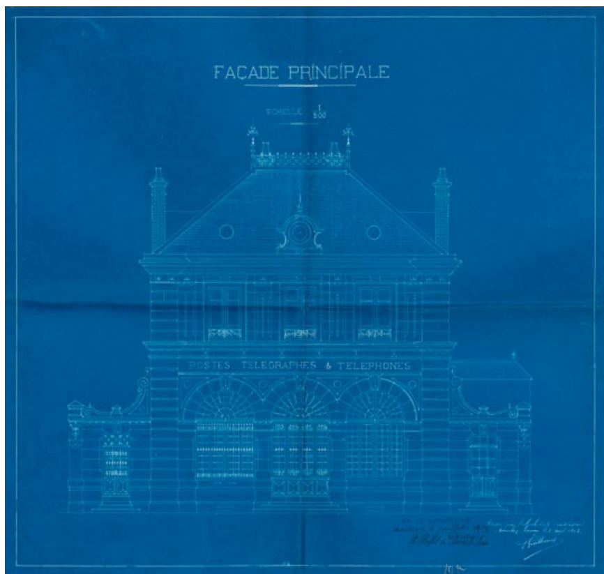
Élévation de la façade antérieure.
