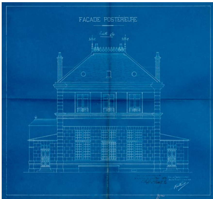
Élévation de la façade postérieure.
