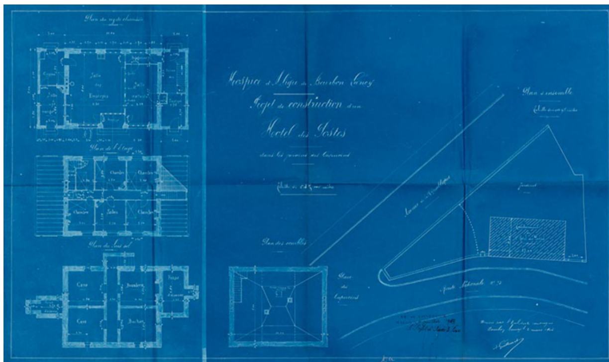
Plan des différents niveaux.
