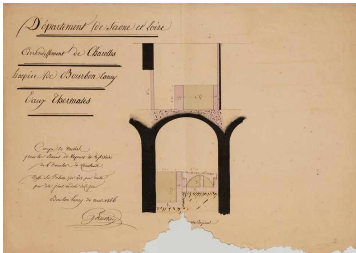
Projet pour la construction d'un bain de vapeur, coupe du rez-de-chaussée et de l'étage (1846).
