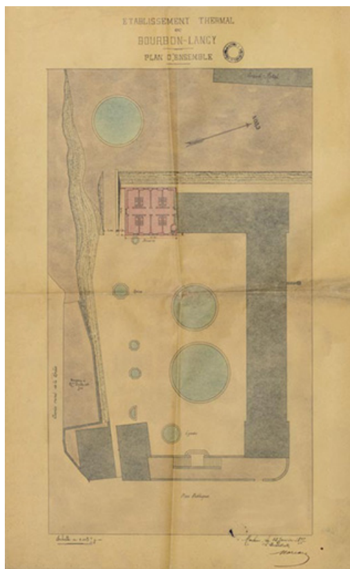
Projet de pavillon annexe, par l'architecte René Moreau (12 janvier 1897), plan de situation. 71, Bourbon-Lancy, 2 Parc thermal
