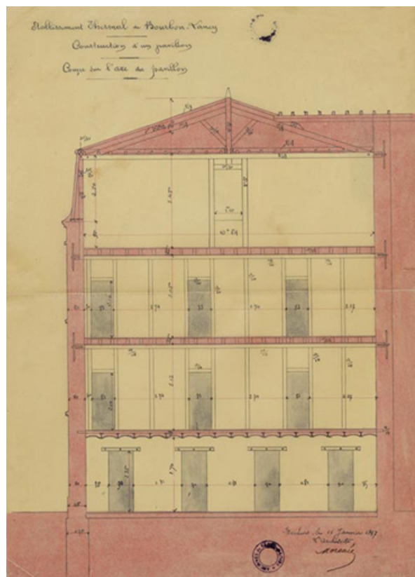
Projet de pavillon annexe, par l'architecte René Moreau (11 janvier 1897), coupe. 71, Bourbon-Lancy, 2 Parc thermal
