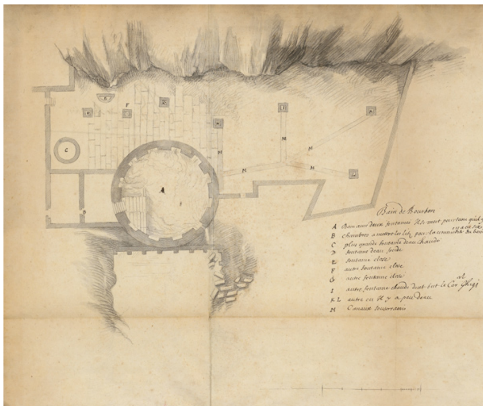
Plan des bains du "Mémoire du traitement fait par la maison du Roy à M. le Cardinal de Chigi" (1664). 71, Bourbon-Lancy, 2 Parc thermal
