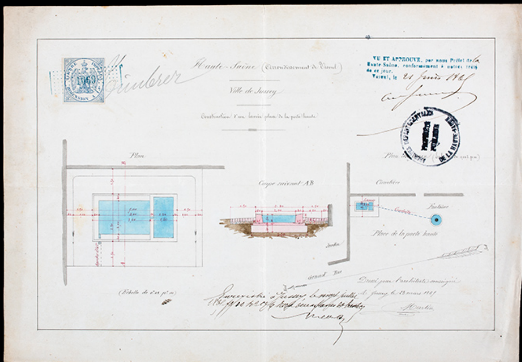
Plan et coupe projetés du lavoir de la porte haute de Jussey, 1865.
