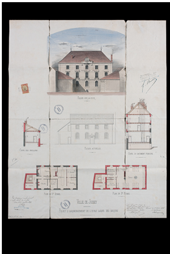
Projet d'agrandissement de l'école laïque de garçons [plans, élévation, coupes], 1879.
