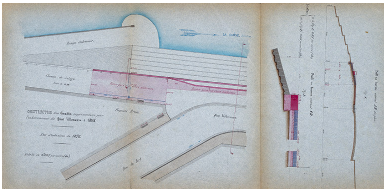
Construction d'un gradin supplémentaire pour l'exhaussement du quai Villeneuve à Gray (1878).
