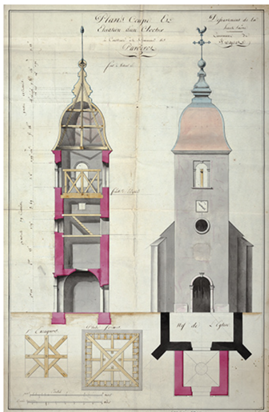
Projet de reconstruction du clocher, 19e siècle. 70, Purgerot Grande Rue
