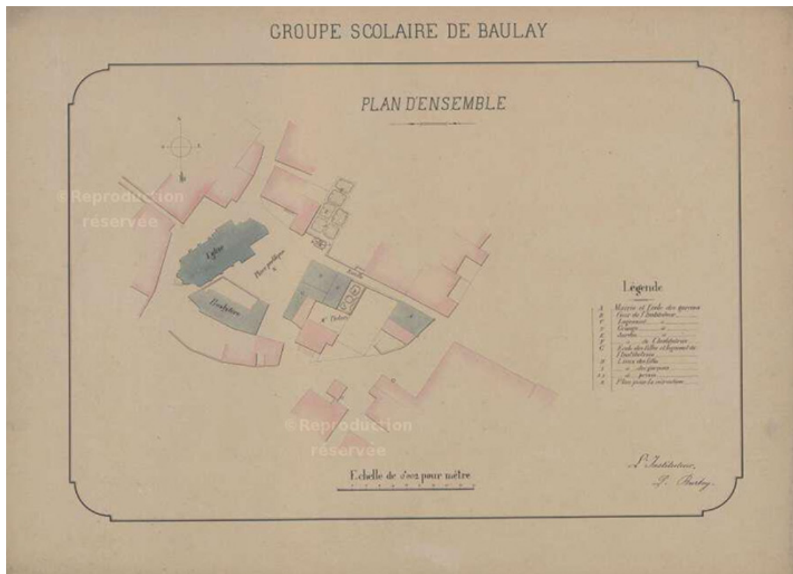
Plan d'ensemble du groupe scolaire de Baulay
