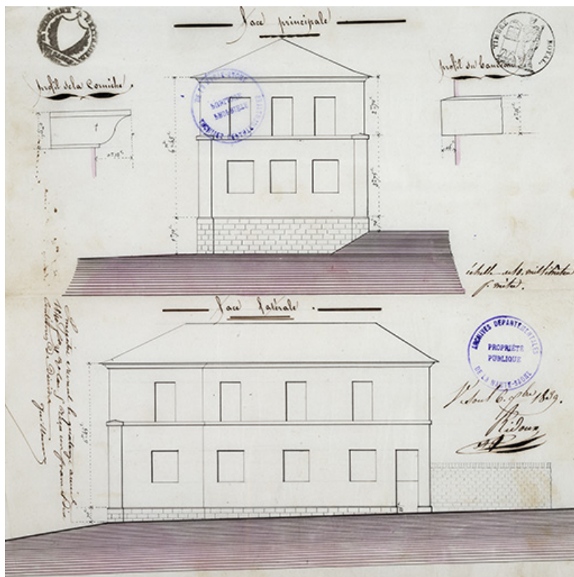
Plans en élévation des façades de la maison commune, 1839
