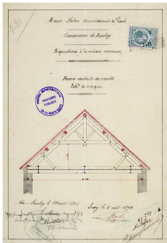
Réparations à la maison commune, plan en coupe de la ferme centrale du comble, 1894 70, Baulay rue de l' Église
