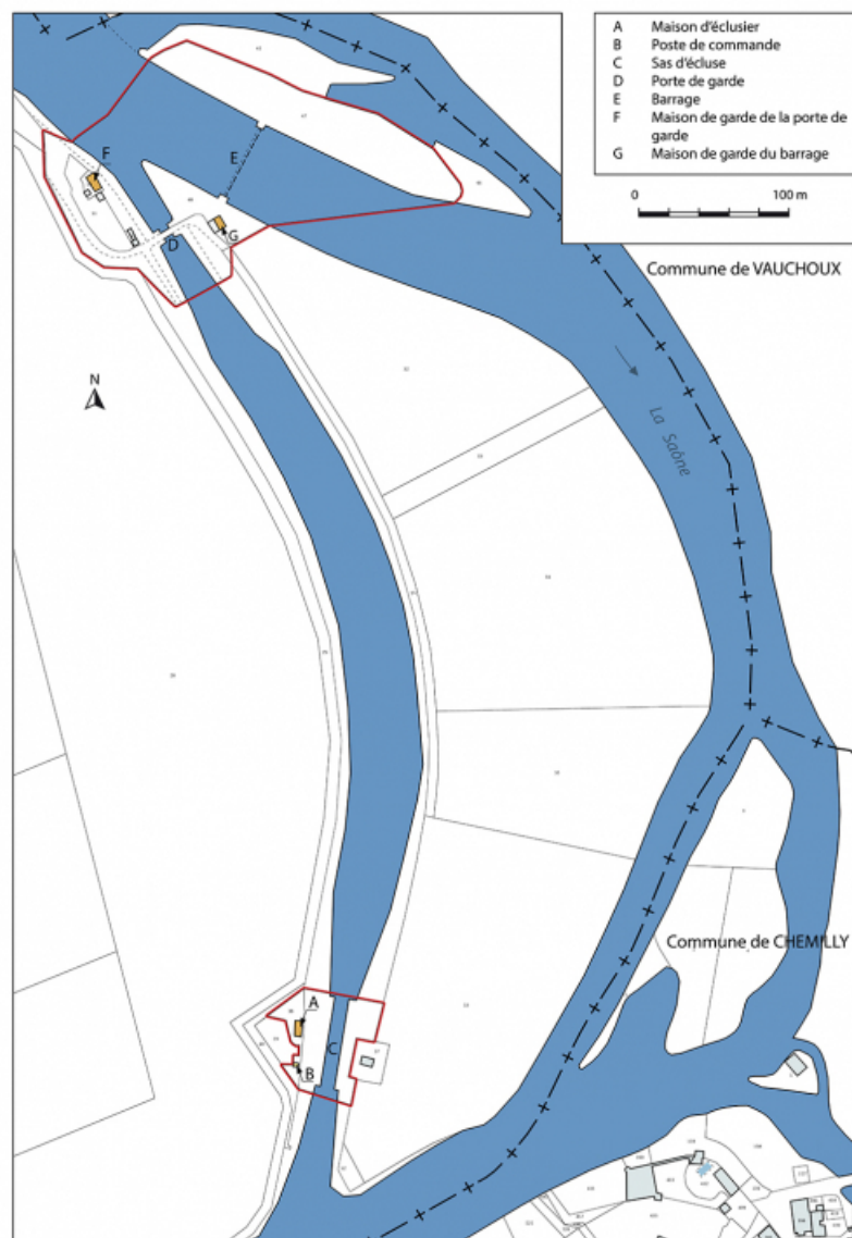
Plan masse et de situation. Détail sud du bief incluant porte de garde et site d'écluse aval. 70, Ferrières-lès-Scey
