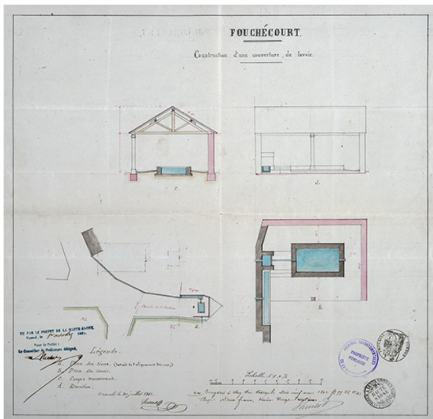
Projet de couverture d'un lavoir (1861).
