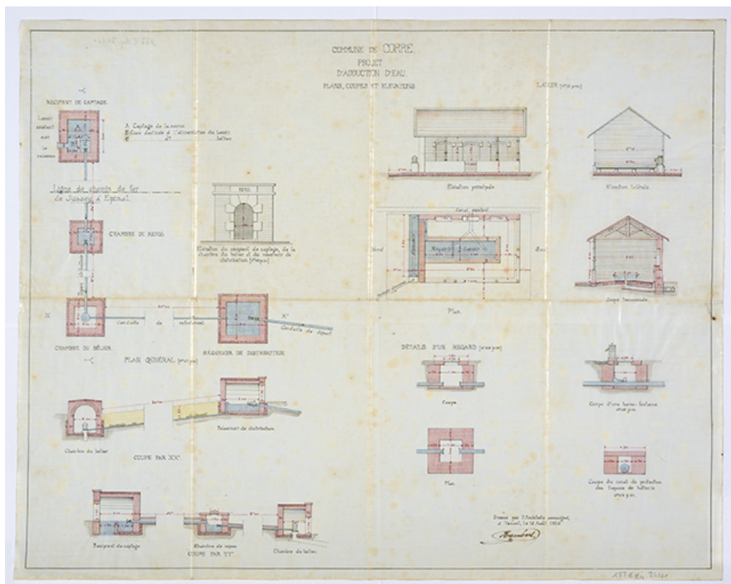
Commune de Corre. Projet d'adduction d'eau. [plans, coupes, élévations.] 1910 70, Corre
