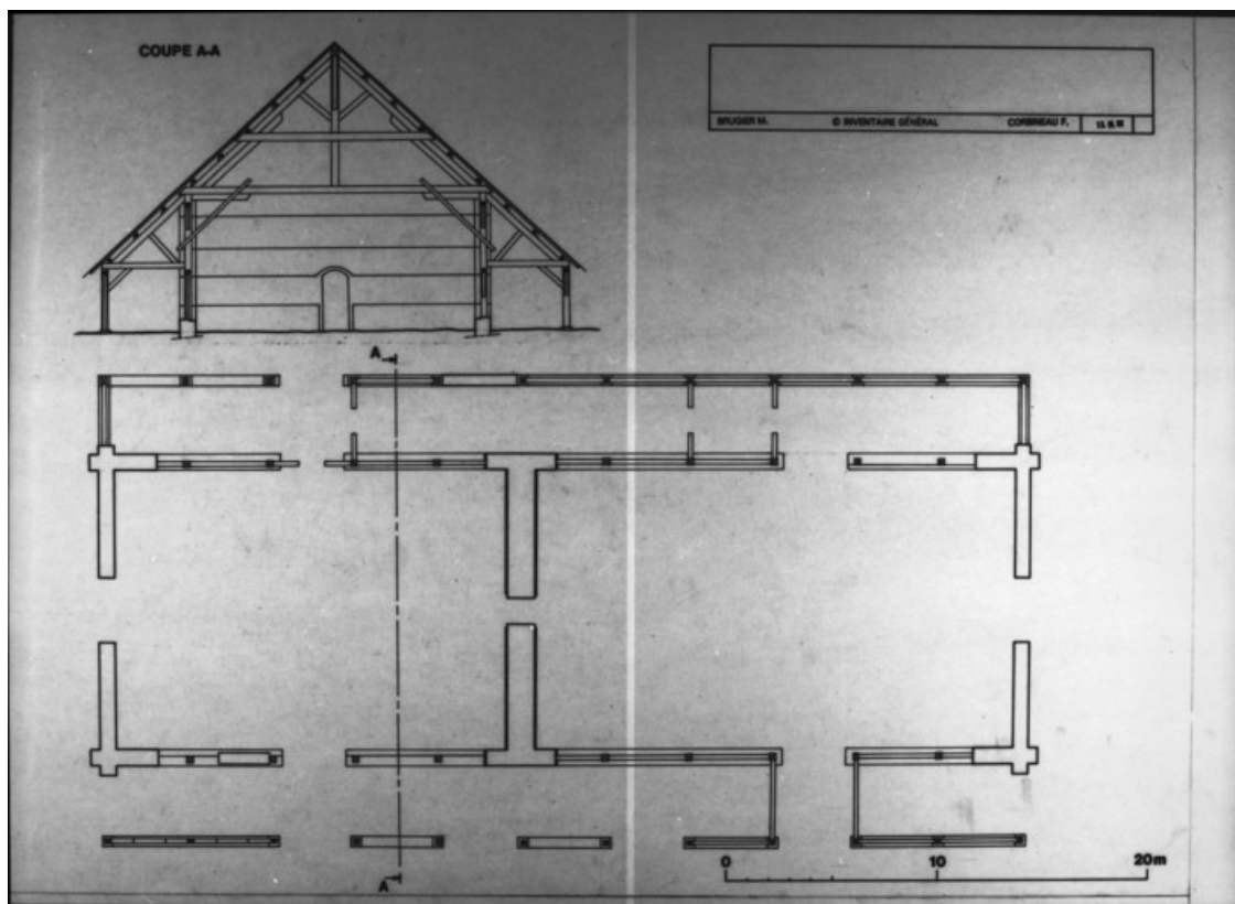
Plan et coupe de la halle à charbon. Relevé graphique, 1988, M. Brugier et F. Corbineau, échelle 1:1250. 70, Beaujeu-Saint-Vallier-Pierrejux-et-Quitteur, lieudit : la Forge
