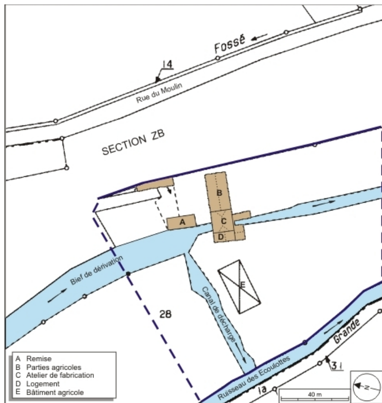
Plan-masse et de situation. Extrait du plan cadastral numérisé, 2008, section ZP, 1:2000 agrandi à 1:1250. Source : Direction générale des Finances Publiques - Cadastre ; mise à jour : 2008.
