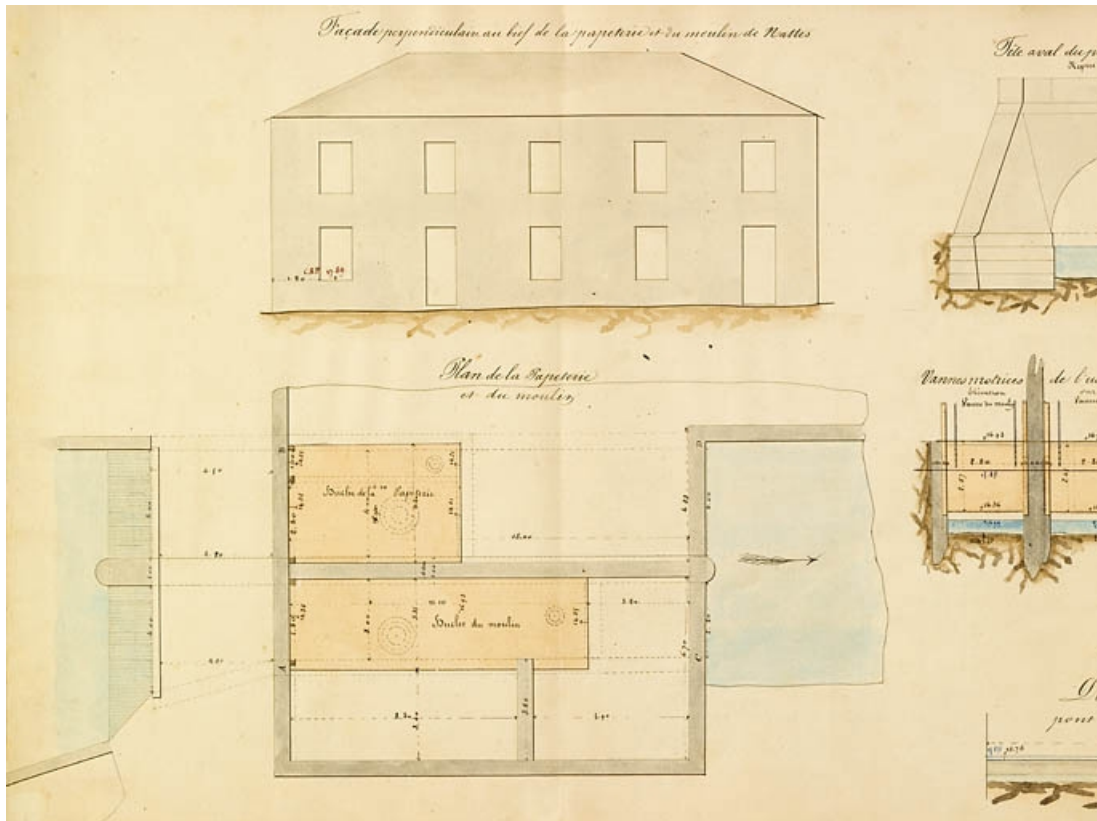
Profils. Plan de la papeterie et du moulin et façade perpendiculaire au bief.
