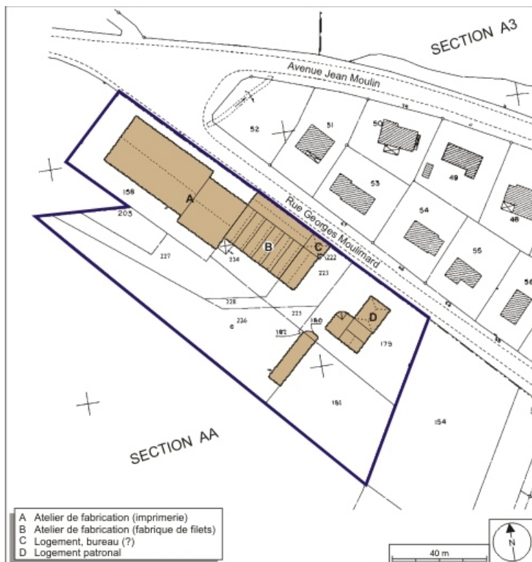
Plan-masse et de situation. Extrait du plan cadastral numérisé, 2008, section AH, 1:1000 réduit à 1:1250. Source : Direction générale des Finances Publiques - Cadastre ; mise à jour : 2008.
