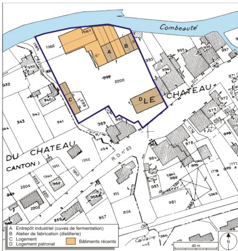
Plan-masse et de situation. Extrait du plan cadastral numérisé, 2008, section E, 1:1250. Source : Direction générale des Finances Publiques - Cadastre ; mise à jour : 2008.
