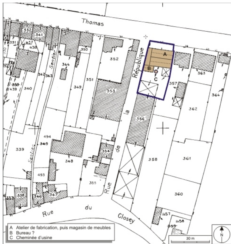
Plan-masse et de situation. Extrait du plan cadastral, 2008, section AI, 1:1000. Source : Direction générale des Finances Publiques - Cadastre ; mise à jour : 2008.
