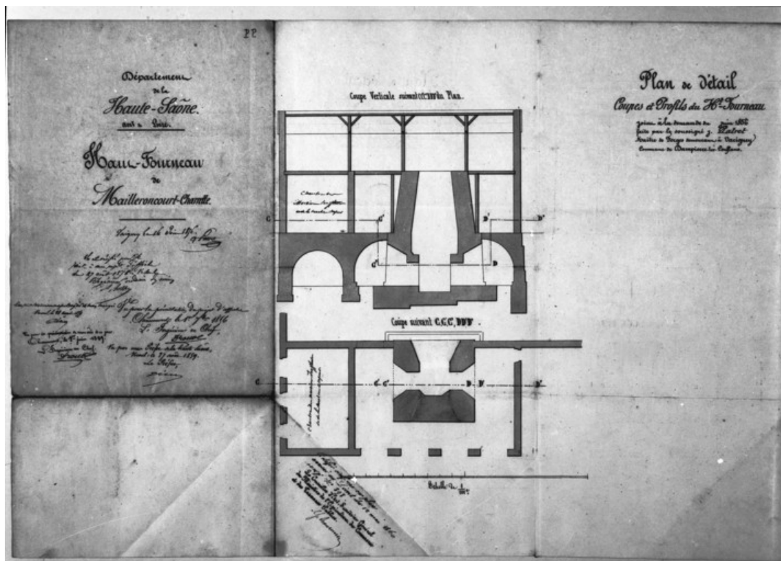
Haut fourneau de Mailleroncourt-Charette. Plan de détail, coupes et profils du haut fourneau.
