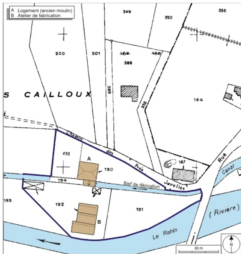
Plan-masse et de situation. Extrait du plan cadastral numérisé, 2008, section AK, échelle 1:1000. Source : Direction générale des Finances Publiques - Cadastre ; mise à jour : 2008.
