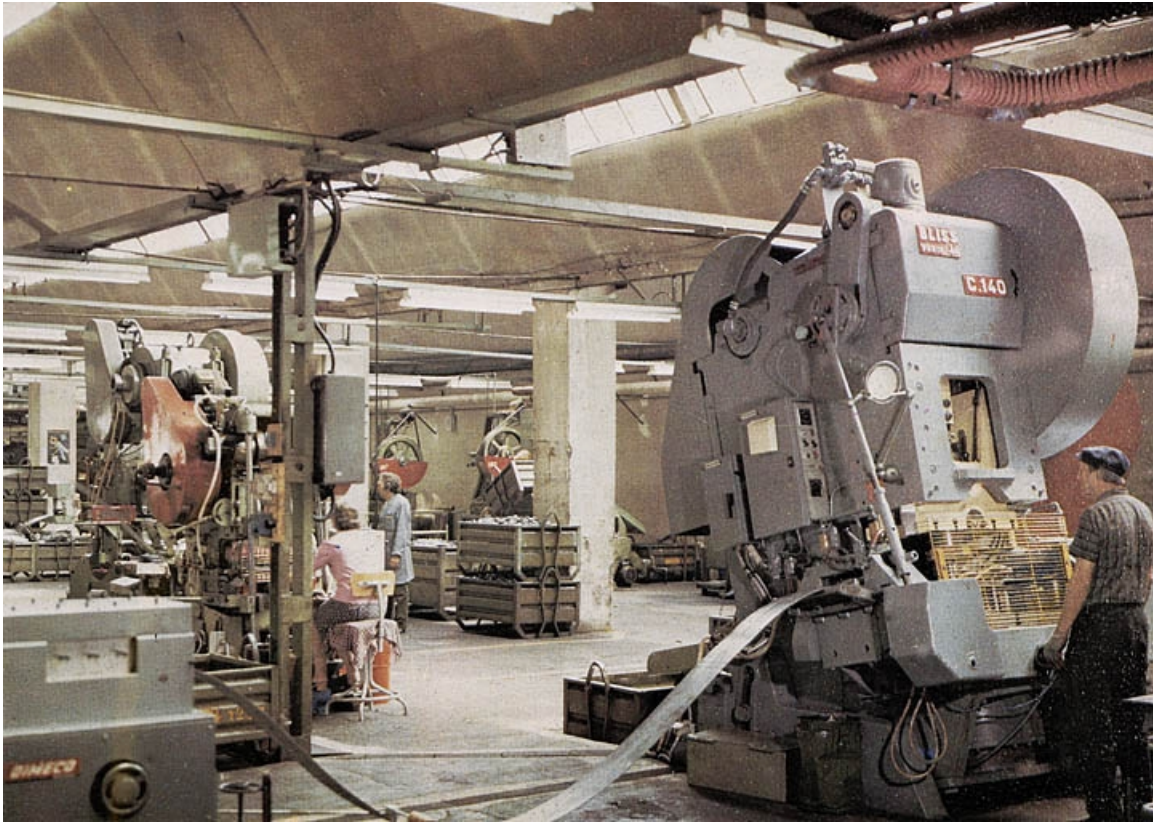
Ensemble de découpage.
