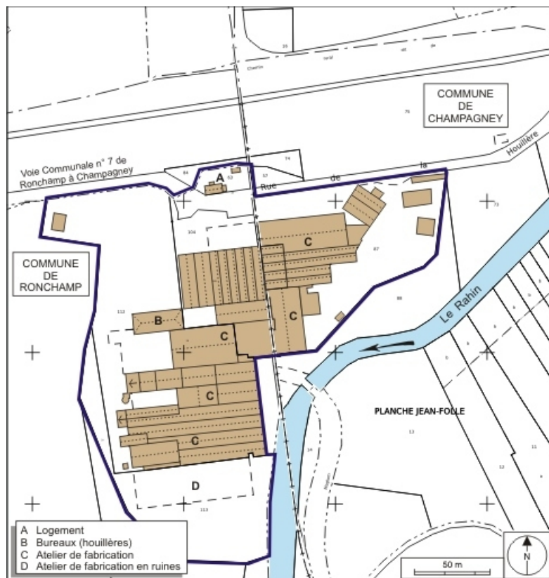
Plan-masse et de situation. Montage d'extraits de plans cadastraux numérisés, 2008, Ronchamp, section AH, 1:1000 et Champagny, section AB, 1:2000, l'ensemble réduit à 1:2000. Source : Direction générale des Finances Publiques - Cadastre ; mise à jour : 2008.
