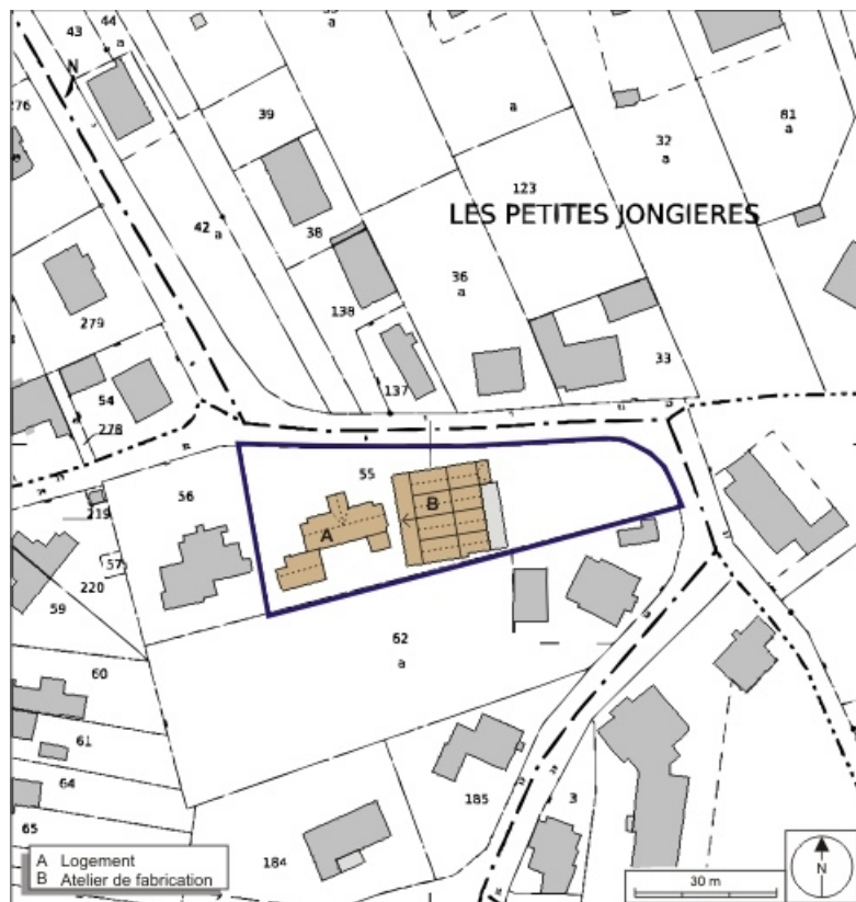
Plan-masse et de situation. Extrait du plan cadastral numérisé, 2008, section AL, échelle 1:1250. Source : Direction générale des Finances Publiques - Cadastre ; mise à jour : 2008.
