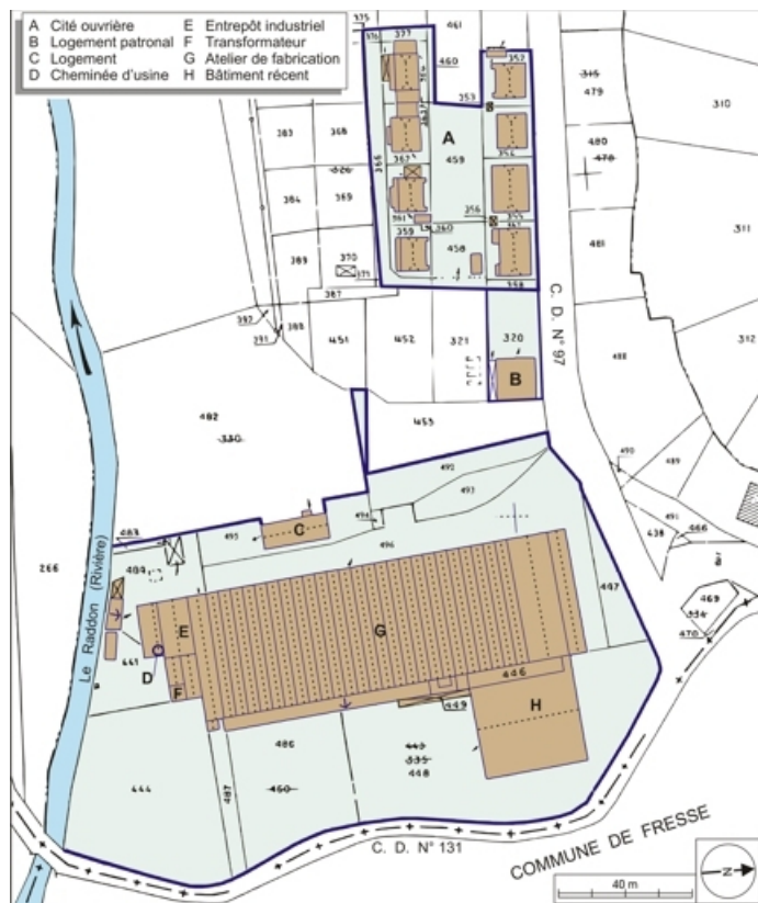
Plan-masse et de situation. Extrait du plan cadastral numérisé, 2005, section B, 1:1000 réduit à 1:1250. 70, Belonchamp, lieudit : le Raddon
