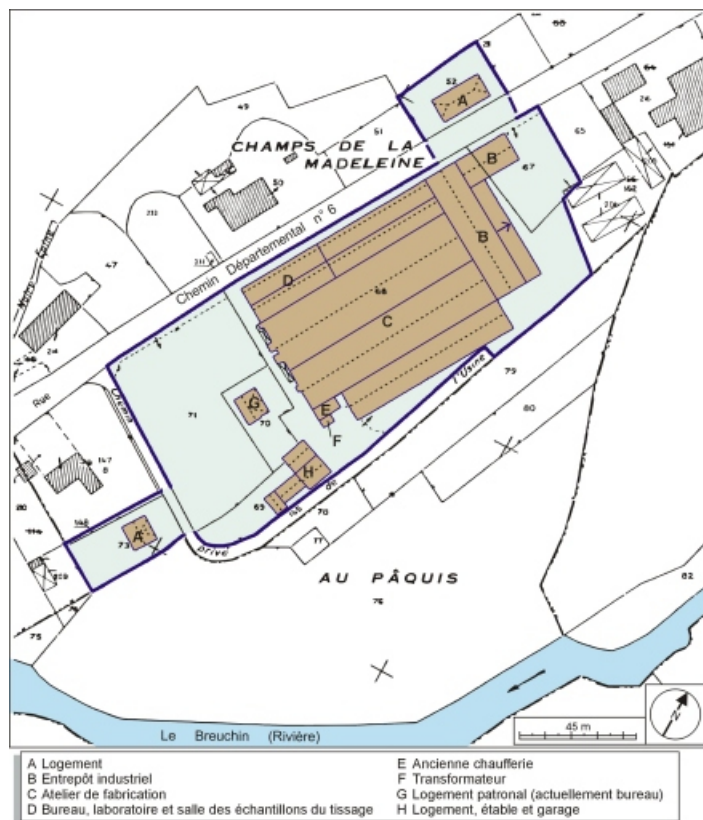
Plan-masse et de situation. Extrait du plan cadastral numérisé, 2005, section AC, 1:1000 réduit à 1:1500. 70, Faucogney-et-la-Mer R.D. 6
