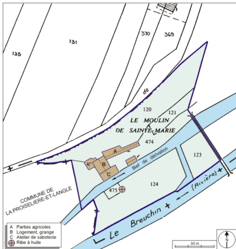
Plan-masse et de situation. Extrait du plan cadastral numérisé, 2005, section A, 1:1250 agrandi à 1:1000. 70, Sainte-Marie-en-Chanois, lieudit : sur le Breuchin
