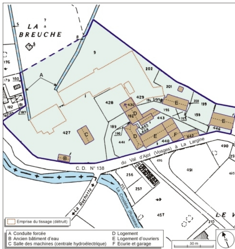
Plan-masse et de situation. Extrait du plan cadastral numérisé, 2005, section AB, 1:1000. 70, La Longine impasse du Tissage
