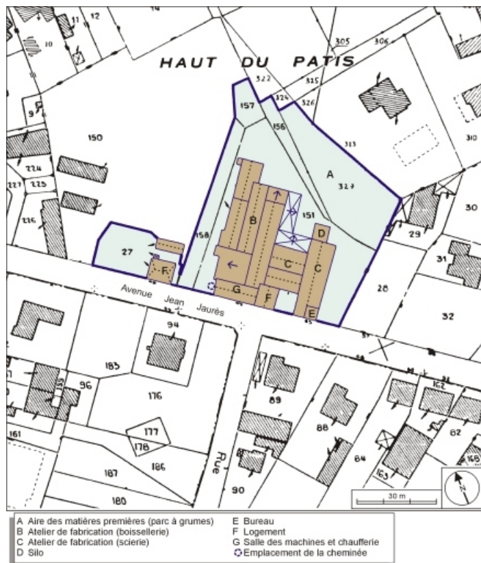
Plan-masse et de situation. Extrait du plan cadastral numérisé, 2005, section AN, 1:1000. 70, Héricourt, 49 à 53 rue Jean Jaurès
